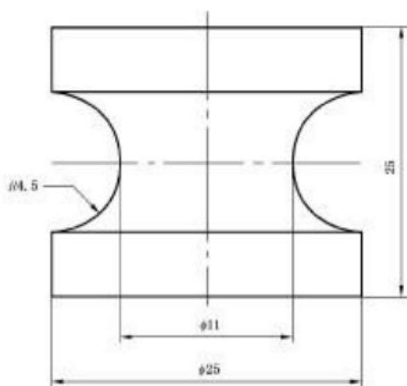
图 3 III型试样
