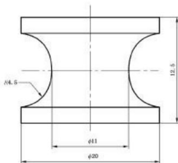
图 2 II型试样
